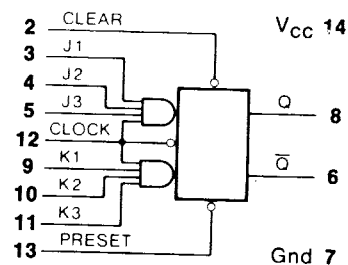
54/7472 J-K Flip-Flop
